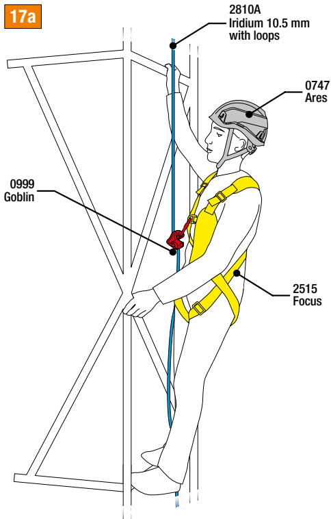
Fig.17a - Dopo la salita del primo operatore è possibile fissare una corda o più corde sulla sommità della struttura, a cui gli operatori possano ancorarsi attraverso opportuni dispositivi anticaduta per corda che permettano la movimentazione verticale.
