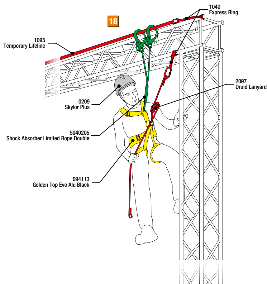
Fig.18 - In caso di strutture metalliche orizzontali, industriali o per lo spettacolo, la progressione può egualmente essere fatta tramite un cordino doppio con assorbitore di energia. Per facilitare la movimentazione è possibile fissare una linea vita temporanea orizzontale lungo la struttura a cui agganciare il cordino (previa verifica di resistenza). Per il posizionamento si suggerisce l'utilizzo di un cordino di posizionamento regolabile.
