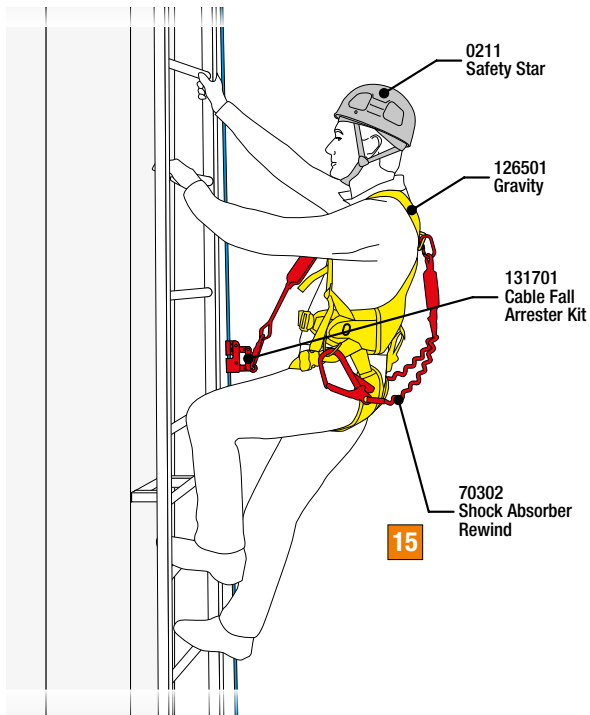
Fig.15 - Molto spesso le strutture metalliche verticali (quali piloni di funivie, pali per turbine eoliche) sono dotati di scale per la progressione abbinata ad un cavo di ancoraggio verticale, su cui installare un dispositivo anticaduta che segua l'operatore durante la movimentazione e intervenga ad arrestare un'eventuale caduta. Per l'ancoraggio nelle zone della struttura prive del cavo verticale, è necessario dotarsi di un cordino doppio con assorbitore di energia.
