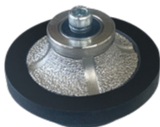
PROFILO "B" CONCAVA
